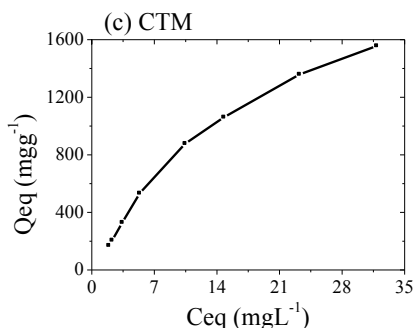
Figura 7. Isothermas de adsorción de Langmuir de amarillo anaranjado para: (a) CCC, (b) CCA y (c) CTM, respectivamente.
