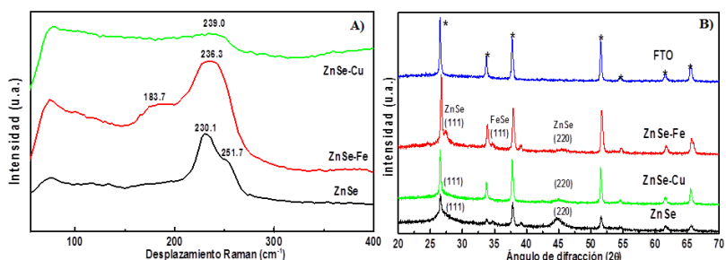
Figura 5. A) Espectro Raman de las películas sintetizadas ZnSe, ZnSe-Fe y ZnSe-Cu B) Patrones de difracción de rayos X para las películas sintetizadas.
